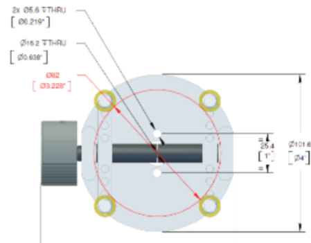
Aufnahmeplatte (unten)
